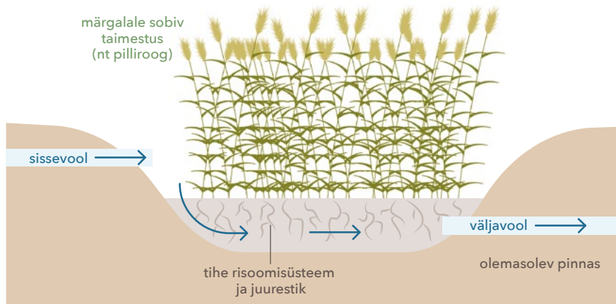
Joonis 46. Horisontaalse veefiltratsiooniga taimeestik-pinnasfilter tehismärgala läbilõige.
