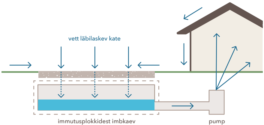
Joonis 23. Näide sademevee kogumise lahendusest läbi vett läbilaskva katendi. Vett saab kasutada majapidamises või näiteks kastmiseks.
