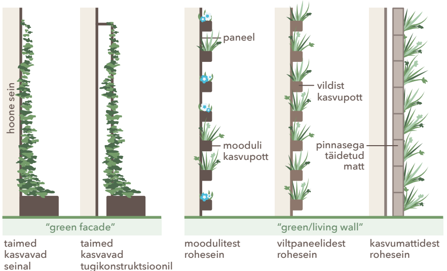
Joonis 18. Erinevat tüüpi roheseinad.
