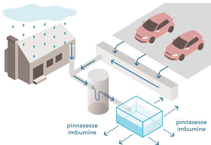
Joonis 21. Imbkaevu tööpõhimõte: sademevesi juhitakse läbi torude ja filterkaevu imbkaevu, kust see imub pinnasesse.
